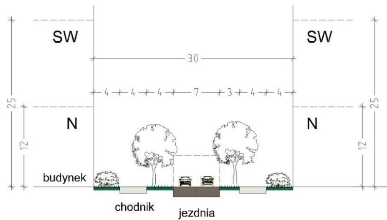
Rys. 7. Model II – wariant z pasami wzdłuż jezdni pod ścianami budynków. Jeśli istnieje możliwość sadzenia drzew przy ulicy (drzewa średnie – II) należy zrezygnować z wprowadzania drzew pod ścianami budynków, a zastąpić je krzewami (bądź pnączami) (wg Borowski i Pstrągowska 2009)
