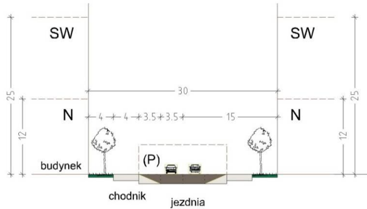
Rys.6. Model II – wariant bez pasa zieleni między chodnikiem a krawędzią jezdni; ulica z drzewami wzdłuż ścian budynków (drzewa najmniejsze – I) (wg Borowski i Pstrągowska 2009)
