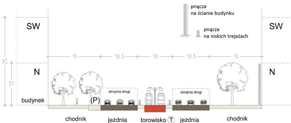
Rys. 8. Model III – wariant z bardzo ograniczonym dostępem do gruntu rodzimego. Możliwe sadzenie jedynie drzew w misach; szerokość ulicy umożliwia zastosowanie dużych drzew (drzewa średnie – II i duże – III), należy je sadzić możliwie jak najdalej od jezdni i od budynków (wg Borowski i Pstrągowska 2009)
